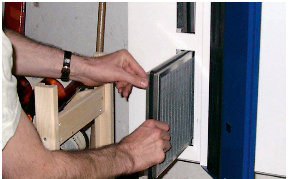
Zustand von Abluft- und Zuluftfilter nach sechs Monaten Betriebszeit (oben); einfacher Filterwechsel: alten Filter herausziehen und den neuen Filter einschieben (rechts)
