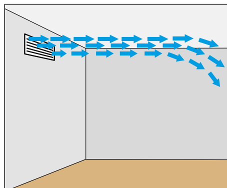
Coanda-Effekt bei Weitwurfelementen: die Luft streicht entlang der Decke weit in den Raum hinein (links).
